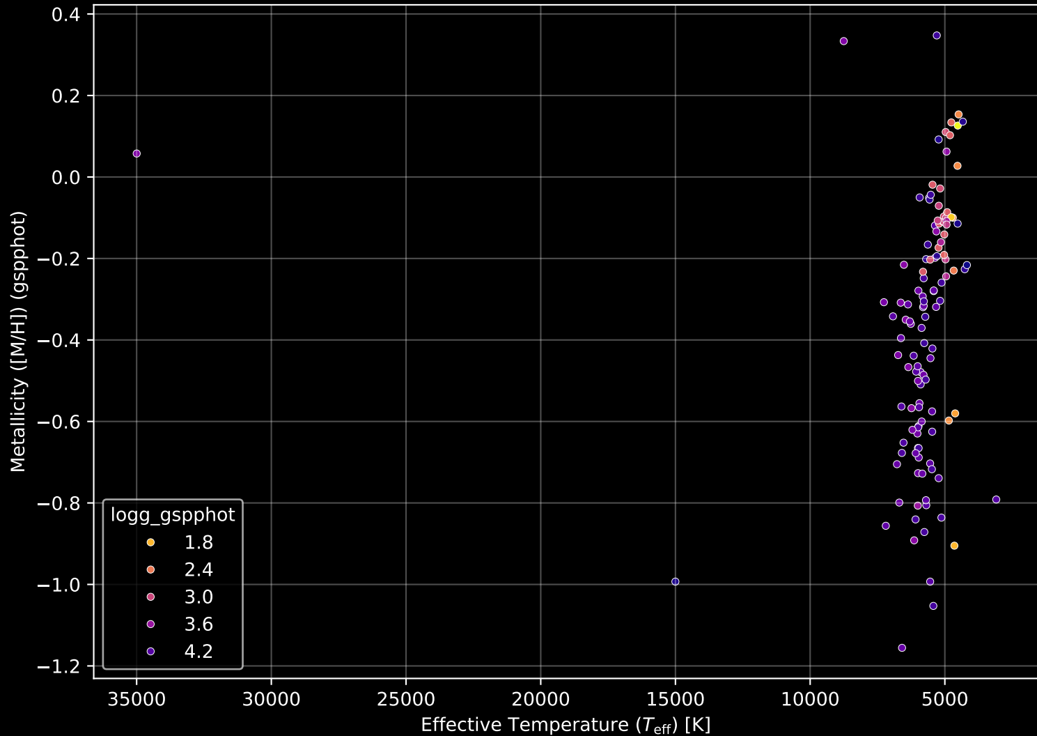
GALAH DR4 Field: [6792] Stellar Population Parameters (n= 125)
