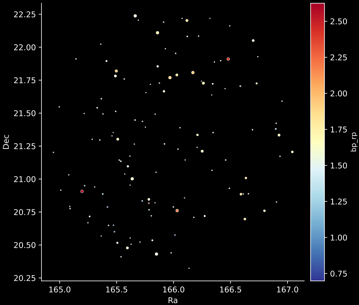
GALAH DR4 Field: [6792] Stars: 125
